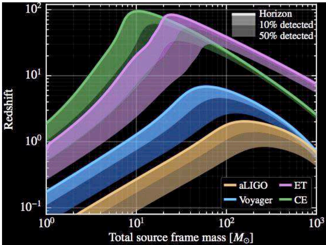
Alcance astrofísico en función de la masa total de los sistemas binarios en coalescencia para distintos futuros detectores. Los contornos sombreados indican el alcance máximo y distancia a la que son observables el 10% y 50% de las fuentes.
