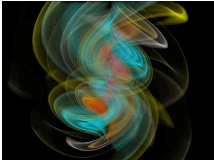
Simulación numérica de la fusión de una binaria de agujeros negros, componentes tridimensionales de la curvatura del espacio-tiempo. Simulación de Sascha Husa y visualización de Rafel Jaume, ambos de la Universidad de les Illes Balears.
