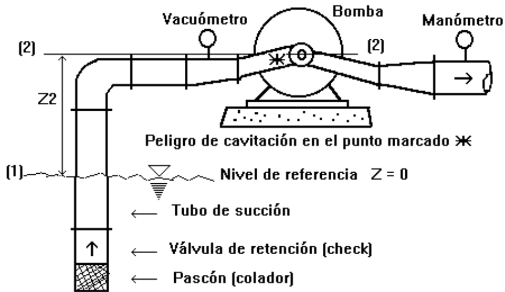
Fig. V.19 - ANALISIS DE LA CAVITACION
