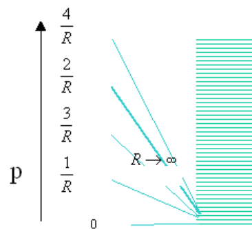
FIGURA 8. Torre de estados de Kaluza-Klein.
