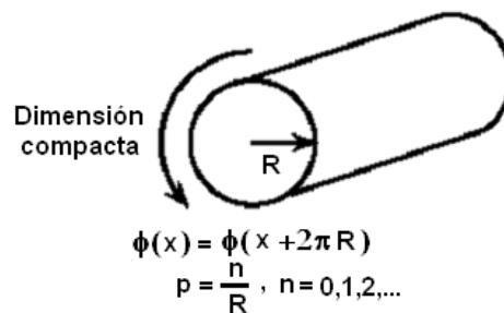
FIGURA 7. El momento en la quinta coordenada es discreto. El campo está sujeto a las condiciones de frontera mostrada.
