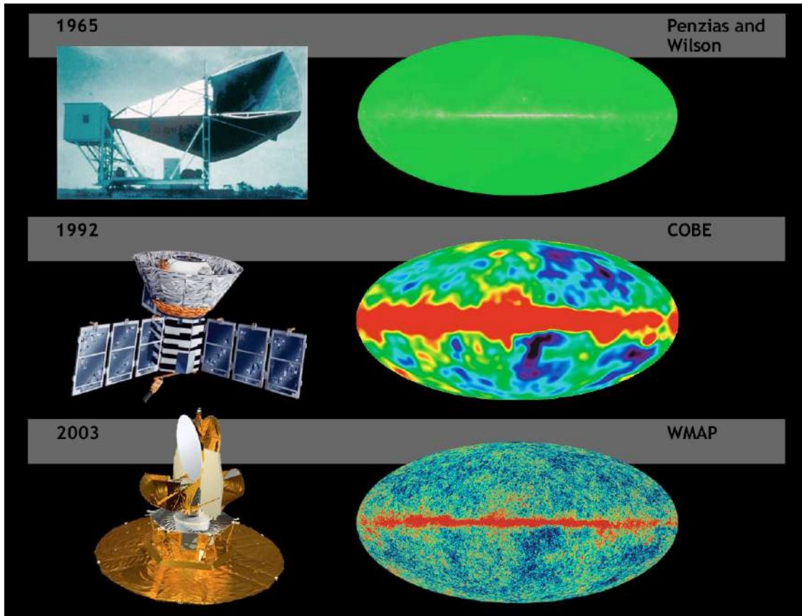
Mapas de la radiación de fondo (Credito: NASA/WMAP Science Team)
